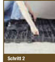
Ganze Lage anlegen und ausrichten
